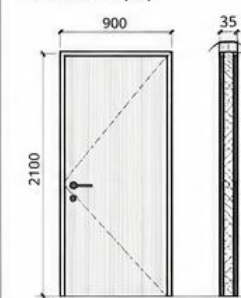
8 DOOR DETAIL SCALE 1:10
