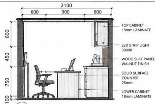
6 SECTION A-A SCALE 1:25
